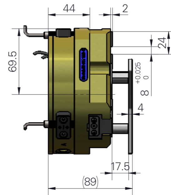
带推料装置图
