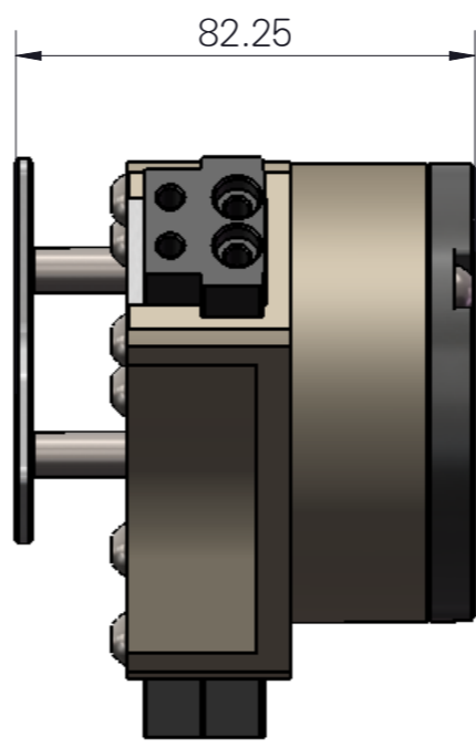
名称: 气动薄款强力夹三爪-D63 型号: FY56N-D63-T-B
