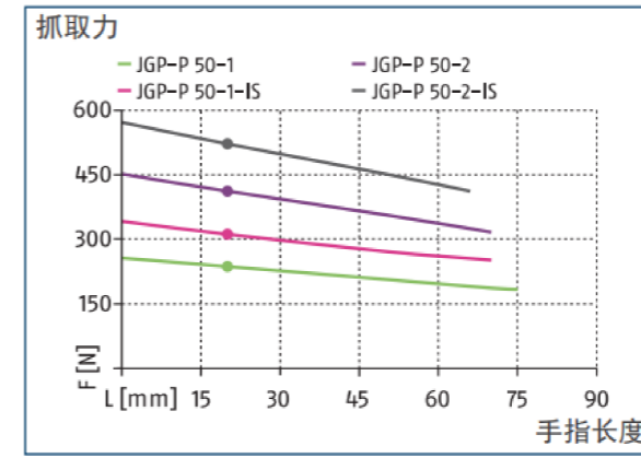
抓取力, 内撑抓取
