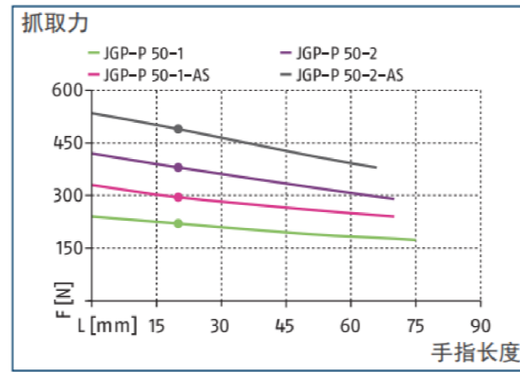
抓取力, 外夹抓取
