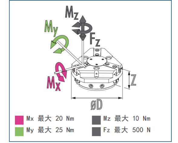
尺寸和最大载荷
