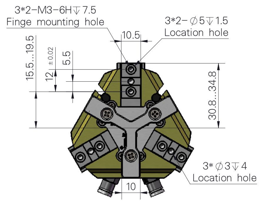
带推料板
