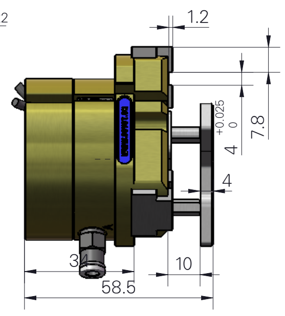
带推料板
