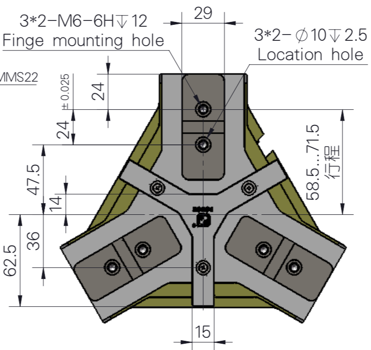
带推料装置图
